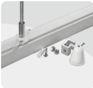
Vario rod suspension EZCLIK (rod length 1m)
